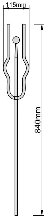
Geländerstab Nr. 1411 Gewicht: 1,6 kg Stab-Material RD 12mm
