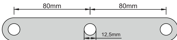
Verbindungsplatte Nr. 1475 Gewicht: 0,2 kg Material: FL 25x6mm
