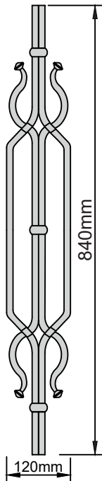
Geländerstab Nr. 1430 Gewicht: 2,8 kg Stab-Material RD 12mm
