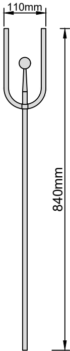
Geländerstab Nr. 1410 Gewicht: 1,3 kg Stab-Material RD 12mm
