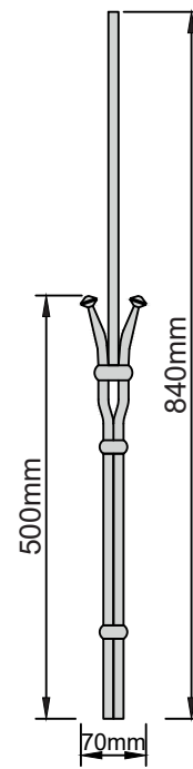
Geländerstab Nr. 1435 Gewicht: 2,0 kg Stab-Material RD 12mm
