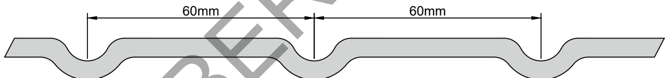
Verbindungsleiste / 1950mm lang Nr. 1448 Gewicht: 2,0 kg Material: FL 25x6mm Maßstab 1:1
