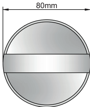
Zierscheibe Eisen Nr. 1470 Gewicht: 0,1 kg Material: 3mm
