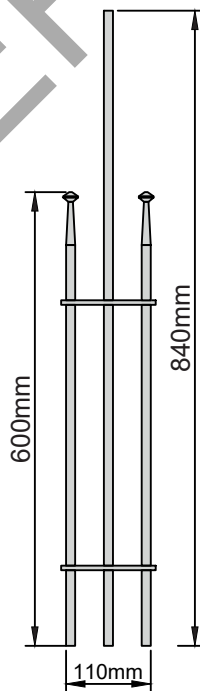
Geländerstab Nr. 1434 Gewicht: 2,0 kg Stab-Material RD 12mm
