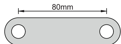
Verbindungsplatte Nr. 1476 Gewicht: 0,1 kg Material: FL 25x6mm
