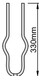
Gitterbügel Nr. 1421 Gewicht: 0,7 kg Stab-Material RD 12mm
