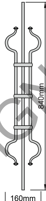
Geländerstab Nr. 1432 Gewicht: 2,2 kg Stab-Material RD 12mm
