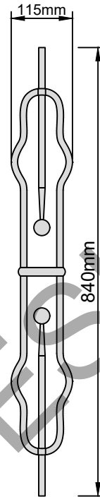
Geländerstab Nr. 1412 Gewicht: 2,2 kg Stab-Material RD 12mm
