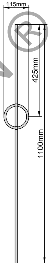
Geländerstab Nr. 1413 Gewicht: 1,5 kg Stab-Material RD 12mm
