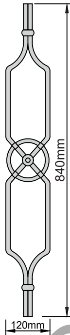
Geländerstab Nr. 1431 Gewicht: 2,0 kg Stab-Material RD 12mm
