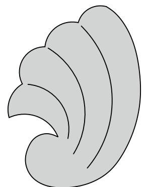
Muschel rechts Nr. 1574-R Gewicht 0,2 kg BL 2mm
