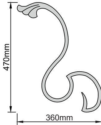
Zierranke Nr. 1534 Gewicht 0,8 kg FL 14x5mm
