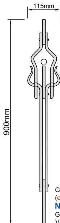
Geländerstab Nr. 1515 Gewicht 2,2 kg VK 12mm
