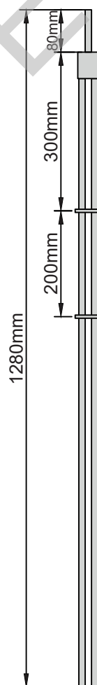
Geländerstütze Nr. 1520 Gewicht 6,0 kg VK 12mm
