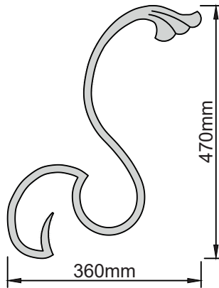
Zierranke Nr. 1535 Gewicht 0,8 kg FL 14x5mm
