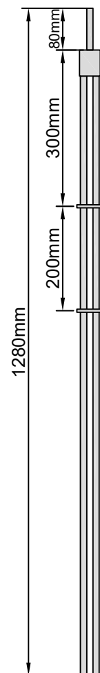
Geländerstütze Nr. 1520 Gewicht 6,0 kg VK 12mm
