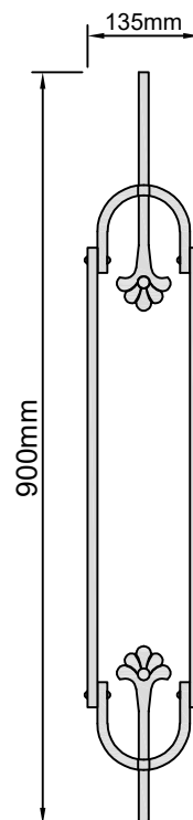
Geländerstab Nr. 1517 Gewicht 2,5 kg VK 12mm
