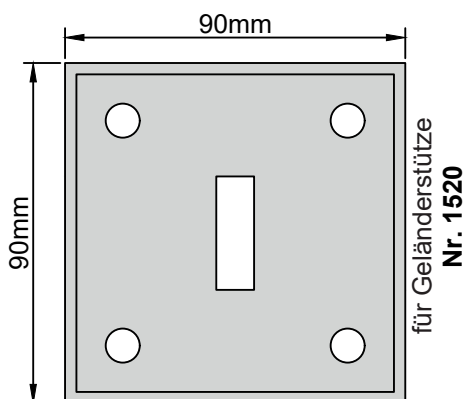
Montageplatte Nr. 1545 Gewicht 0,6 kg Material: 5mm, FL 30x10mm
