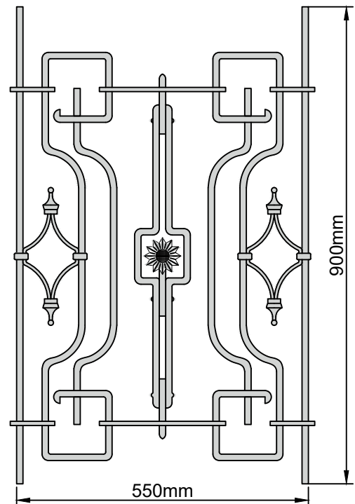
Mittelstück Nr. 1531 Gewicht 11,0 kg VK 12mm
