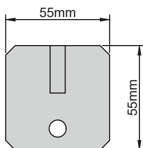
Montagewinkel Nr. 1546 Gewicht 0,2 kg Material: 5mm, FL 25x8mm
