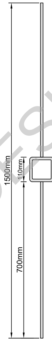
Balkongeländerstab Nr. 1524 Gewicht 2,0 kg VK 12mm
