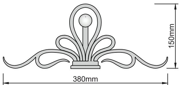
Aufsatzverzierung (ohne Kugel) Nr. 1538 Gewicht 0,9 kg FL 12x6mm / 10x3mm, RD 10mm
