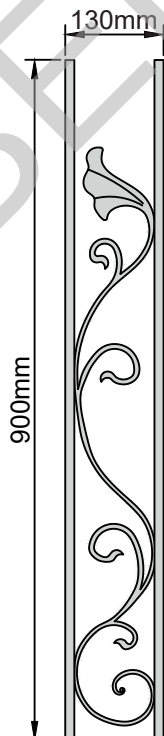
Seitenteil Nr. 1533 Gewicht 3,2 kg VK 12mm, FL12x6mm ohne Vierkant Nr. 1533-oV Gewicht 1,0 kg
