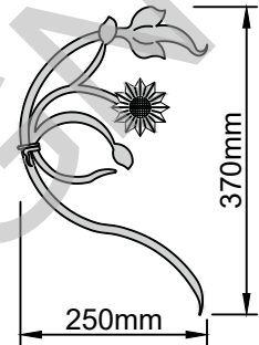
Zierranke Nr. 1526 Gewicht 0,8 kg RD 10mm
