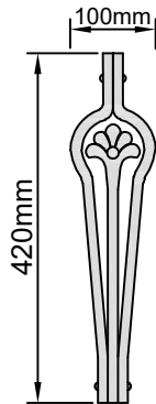
Geländerstab Nr. 1563 Gewicht 1,5 kg VK12mm
