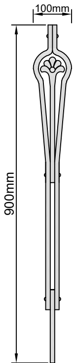
Geländerstab Nr. 1562 Gewicht 2,5 kg VK12mm
