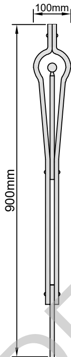
Geländerstab (ohne Kugel) Nr. 1564 Gewicht 2,5 kg VK12mm
