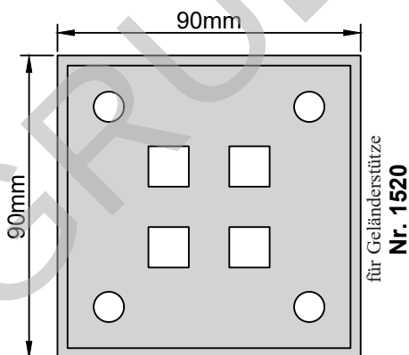
Bodenplatte Nr. 1547 Gewicht 0,3 kg Material: 5mm
