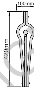
Geländerstab (ohne Kugel) Nr. 1565 Gewicht 1,5 kg VK12mm
