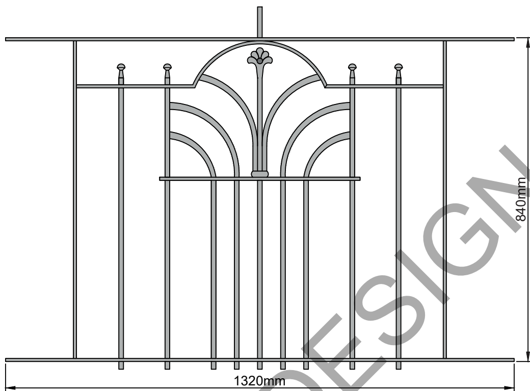
Nr. 1656-VA Edelstahl K240 geschliffen
