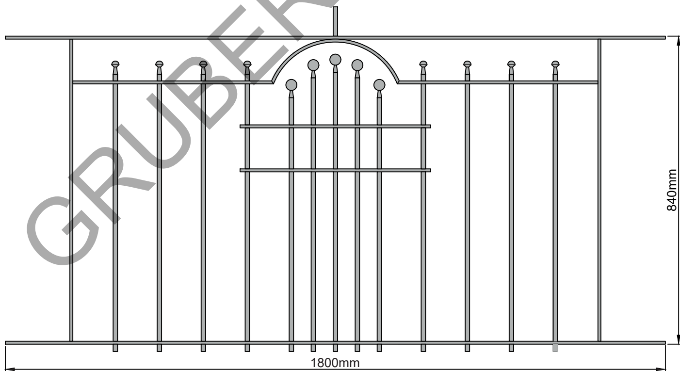
Nr. 1655-VA Edelstahl K240 geschliffen
