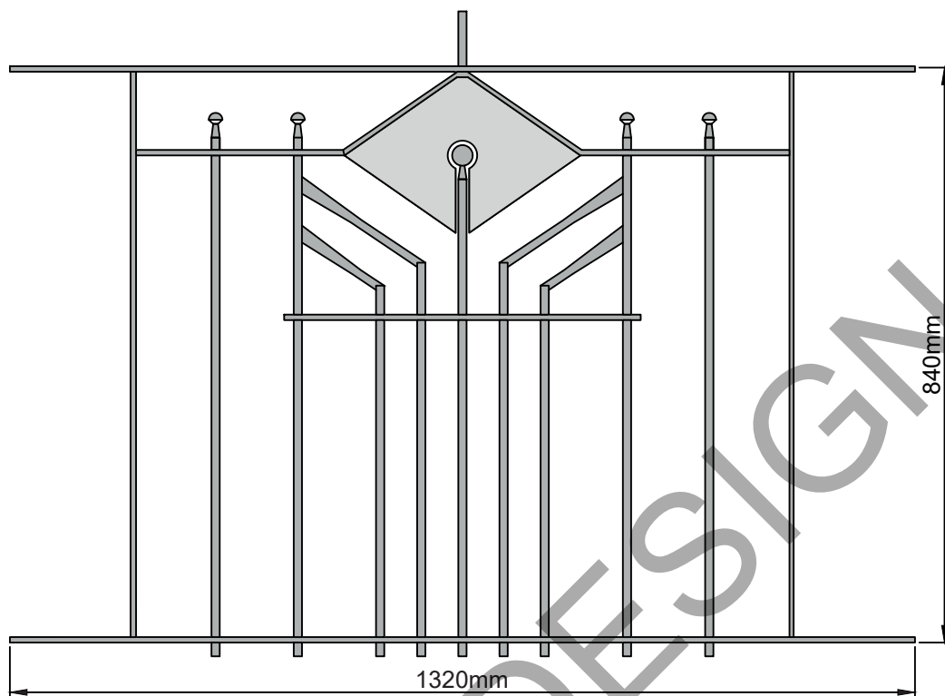
Nr. 1650-VA Edelstahl K240 geschliffen
