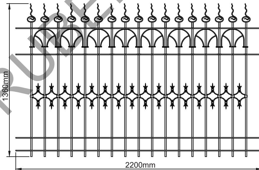
Zaunfeld Nr. 1771 Gewicht 59,5 kg VK 14mm, FL 25x8mm
