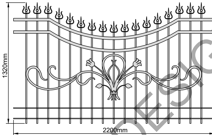
Zaunfeld Nr. 1772 Gewicht 53,5 kg VK 14mm, FL 25x8mm
