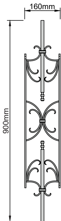
Geländerstab Nr. 1716 Gewicht 3,3 kg VK 14mm, FL 15x5mm
