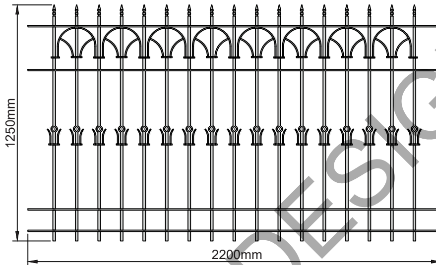
Zaunfeld Nr. 1770 Gewicht 58,0 kg VK 14mm, FL 25x8mm
