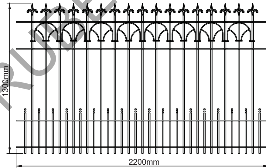
Zaunfeld Nr. 1775 Gewicht 67,5 kg VK 14mm, FL 25x8mm
