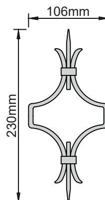
Distanzelement Nr. 1727 Gewicht 0,35 kg FL 15x6mm Maßstab 1:5
