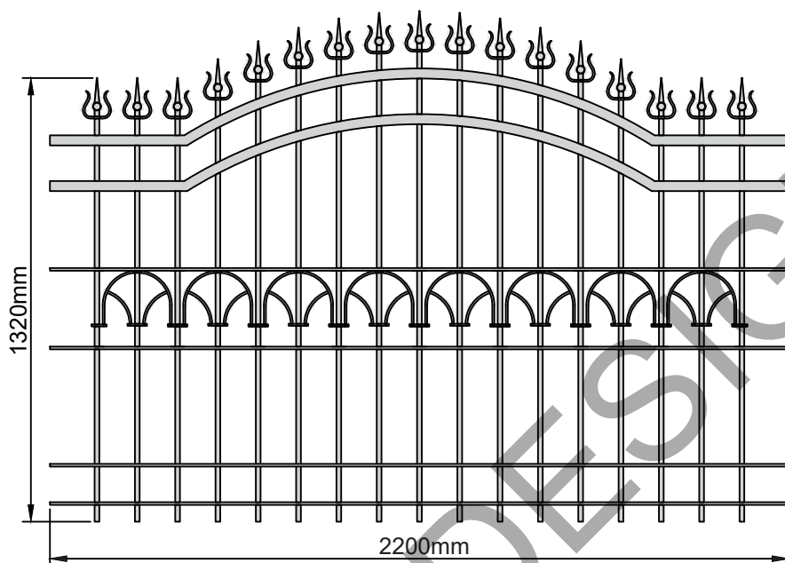
Zaunfeld Nr. 1776 Gewicht 55,0 kg VK 14mm, FL 25x8mm
