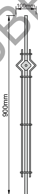
Geländerstab Nr. 1719 Gewicht 2,7 kg VK 14mm, FL 15x6mm
