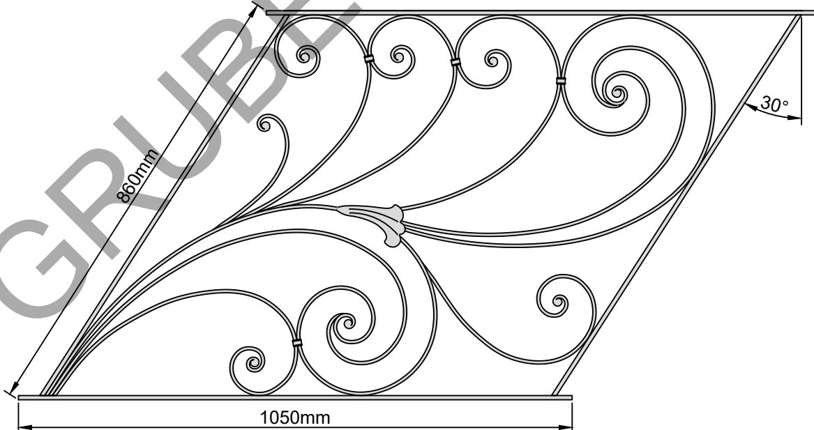
Mittelstück Schräg 30 Grad - Li+Re verwendbar Nr. 1735 Gewicht 12,5 kg FL 25x8mm, FL 15x6mm
