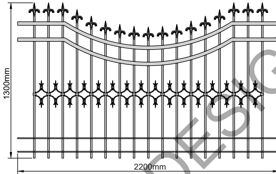
Zaunfeld Nr. 1774 Gewicht 49,5 kg VK 14mm, FL 25x8mm
