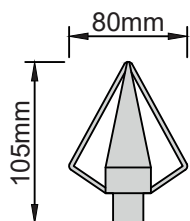
Diamantspitze Nr. 1726 Gewicht 0,25 kg Maßstab 1:5
